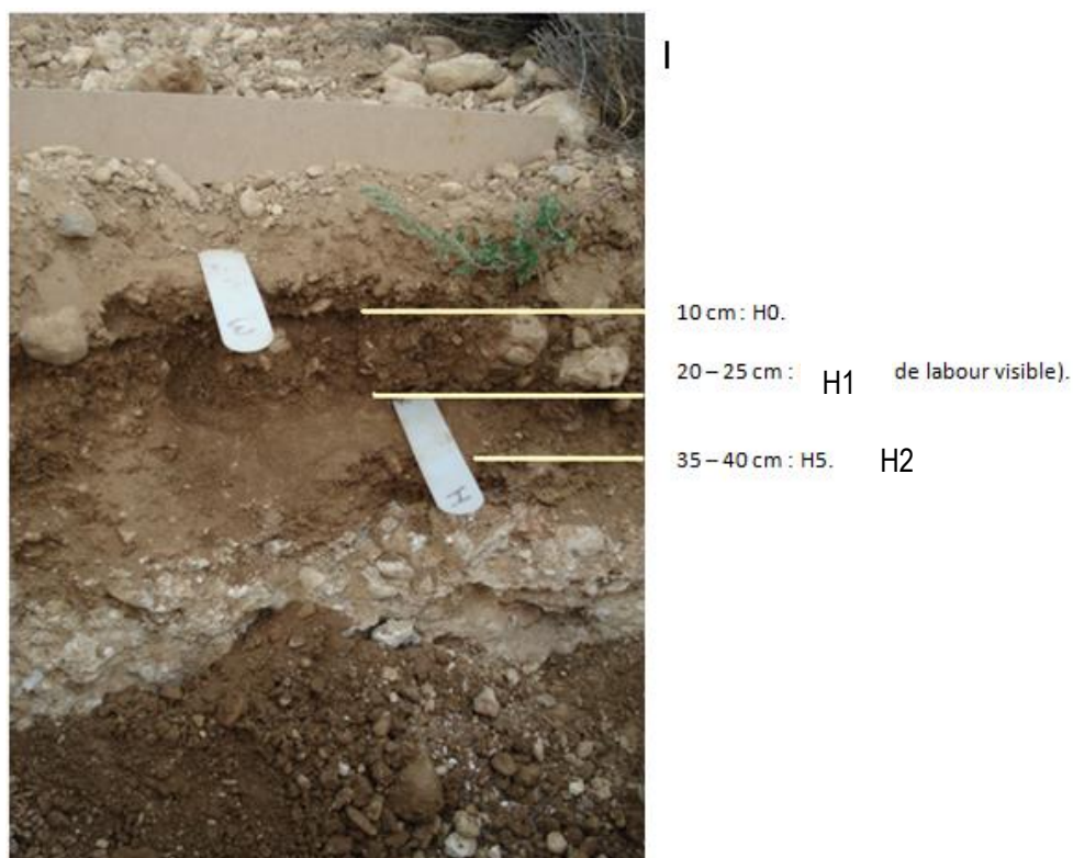
Figure 7 : Exemple de profil cultural sous lavandin sur sol superficiel (<40 cm) sans dégradation majeure
