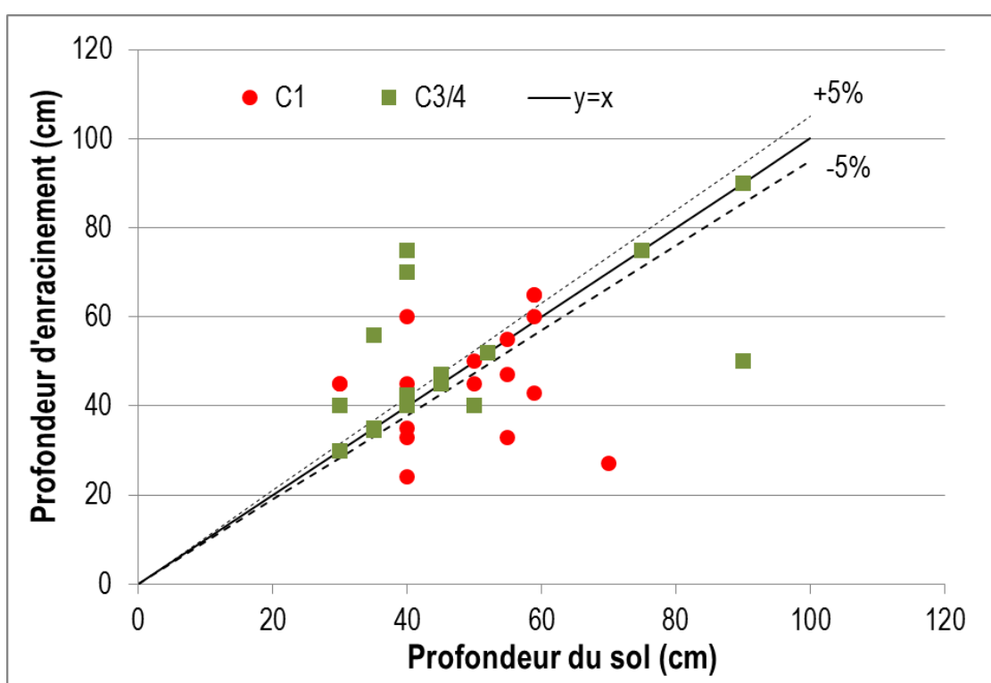
Figure 20 : Relation entre profondeur d'enracinement et profondeur de sol, avec identification des âges de coupe
